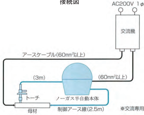
接続図
